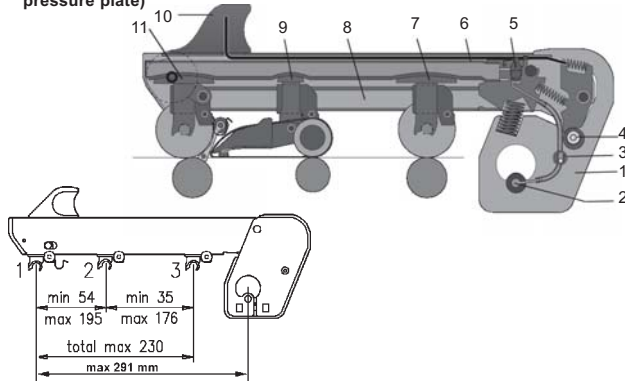
Fig. A: Weighting arm PK 6000-1252 924
